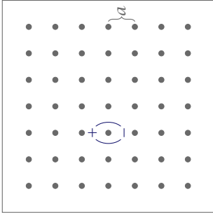
Frenkel
