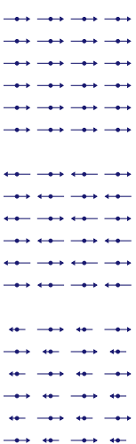
► 5.4 Skizze der drei Grundformen des Ferromagnetismus. Ganz links der Ferromagnetismus, in der Mitte der Antiferromagnetismus und rechts der Ferrimagnetismus. Für eine Erklärung siehe Text. Nach Hunklinger [2].
